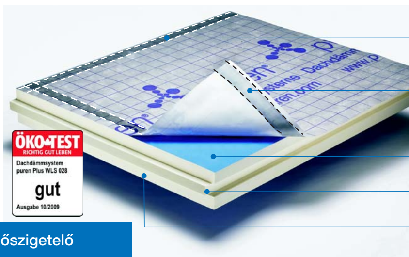
puren Plus tetőszigetelő rendszer: felső oldali 4 cm széles dupla ragasztás
